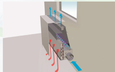
WAND INDUCTIE-UNITS
