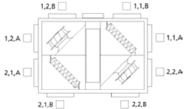
Ventilator positie 1 - Uitvoering rechts
