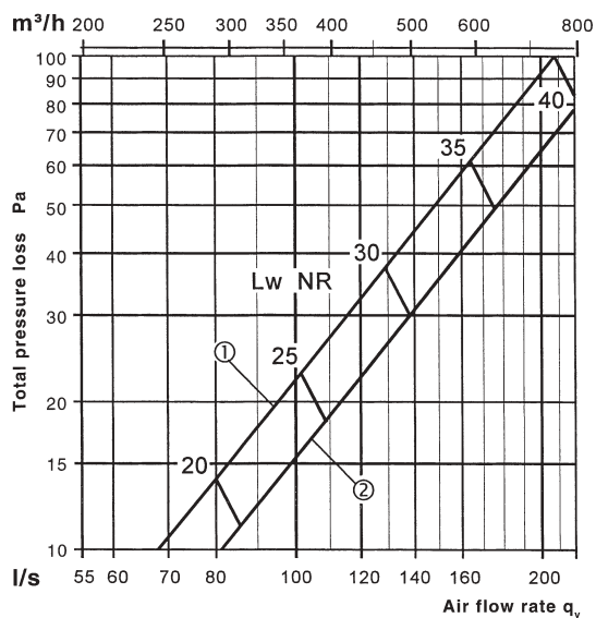
Fig. 6 - WKA 155/45, one way blow
